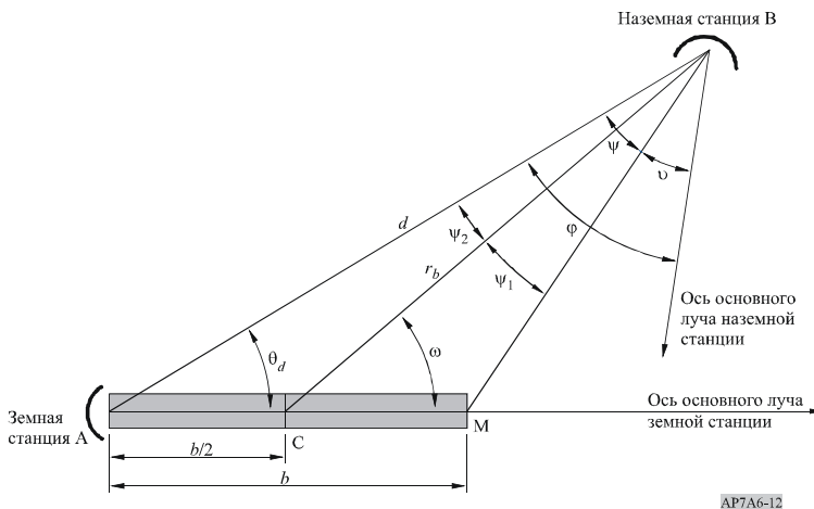
РИСУНОК 12 Геометрия распространения в горизонтальной плоскости
