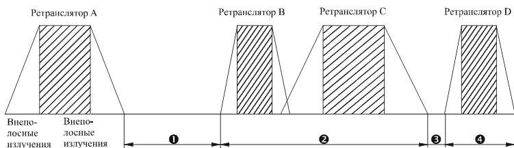
РИСУНОК 2 Пример применимости предельных уровней излучений в области побочных излучений в области спутникового ретранслятора
